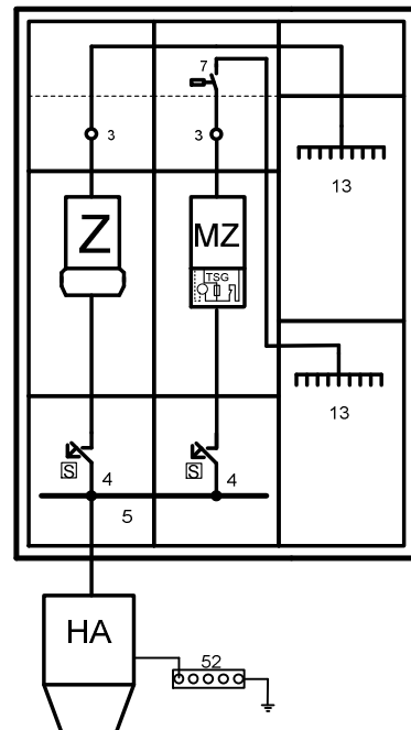
P 1.06 Einkundenanlage mit Freigabe- steuerung (Einfamilienhaus)
